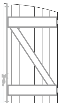
Barres et écharpes avec cintre découpé sans emboîture
