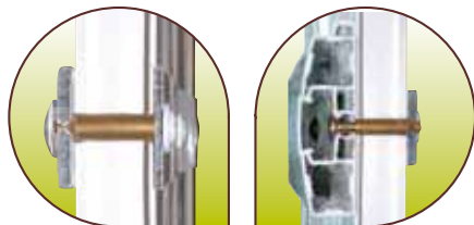
Visserie de sécurité anti-effraction
