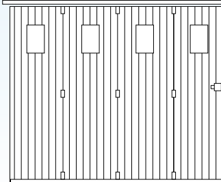
4 vantaux ouverture à déplacement latéral (PDL) en 26 mm avec option hublots
