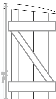
Barres et écharpes avec cintre découpé sur emboîture en biais
