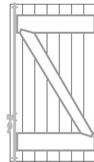
Barres avec écharpe entaillée
