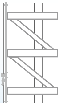
Double barres et écharpes type 1
