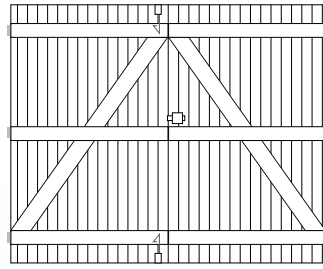
2 vantaux ouverture extérieure à barres et écharpes (PBEI) en 26 ou 32 mm
