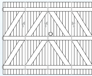
4 vantaux à barres et écharpes ouverture extérieure en 26 ou 32 mm
