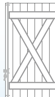
Barres et écharpes croisées
