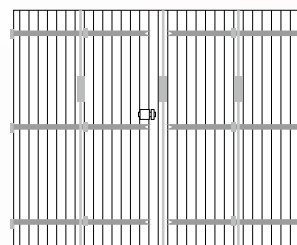
Porte de garage à 4 vantaux à pentures et contre-pentures (PC3) ouverture intérieure ou extérieure en 28 mm présentée avec l'option pentures queue de carpe.
