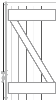
Barres et écharpes emboîture haute
