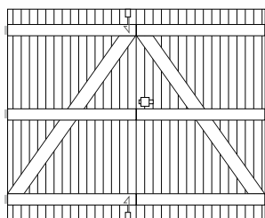
Porte de garage à 2 vantaux ouverture extérieure à barres et écharpes (PBEI) en 28 mm.
