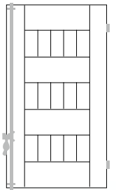
Volet à cadre rapporté avec deux traverses intermédiaires
