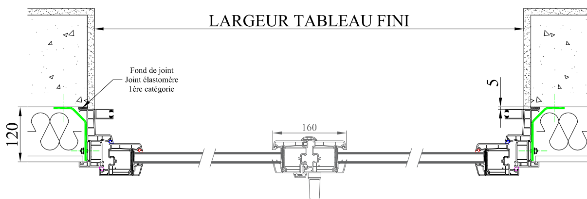
COUPE HORIZONTALE
