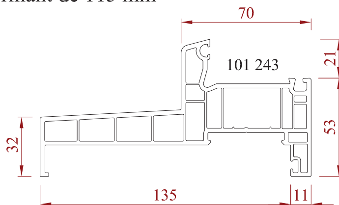
Dormant de 135 mm
