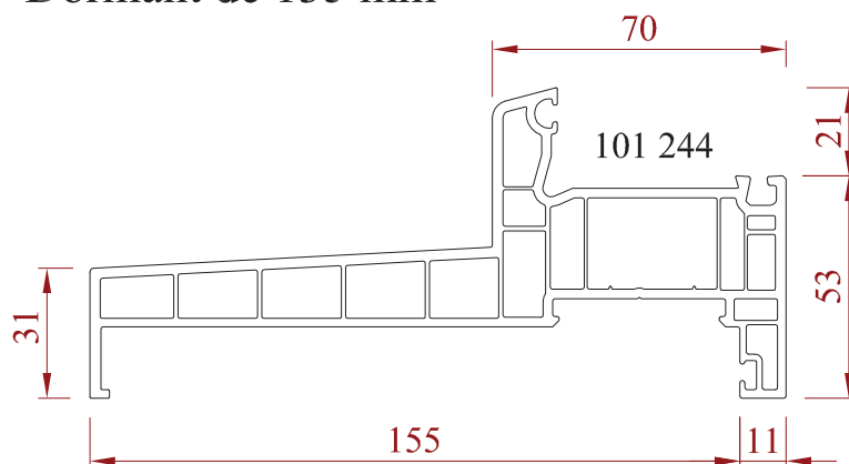
Dormant de 155 mm
