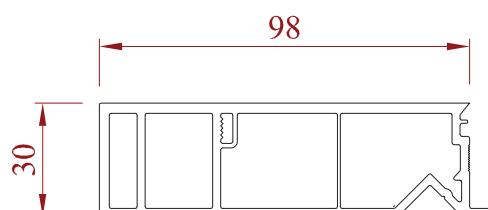
Tapée de 98 mm
