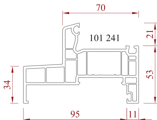
Dormant de 95 mm
