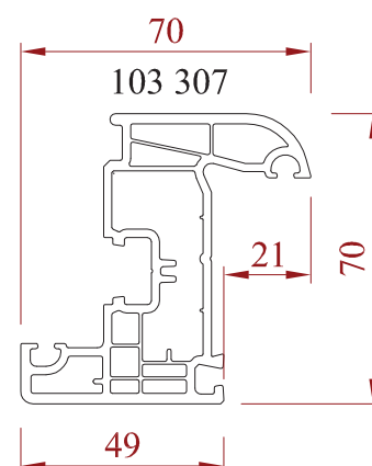
Ouvrant de fenêtre
