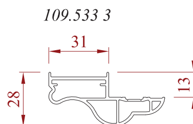
Habillage mouluré (13 mm)
