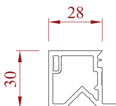
Tapée de 28 mm
