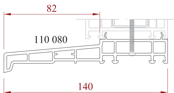
Pièce d'appui de 140 mm
