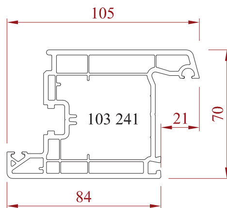
Ouvrant de porte d'entrée
