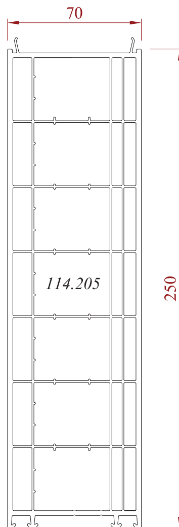
Elargisseur de 250 mm
