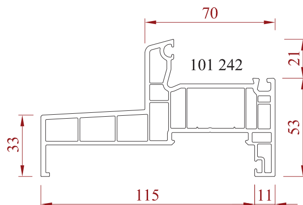
Dormant de 115 mm
