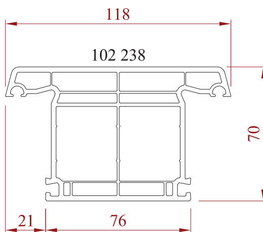
Traverse / Meneau de 118 mm
