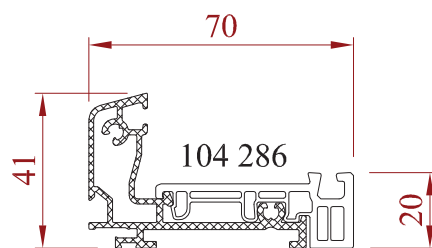
Seuil alu de 41 mm
