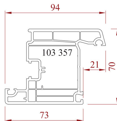
Ouvrant de porte-fenêtre
