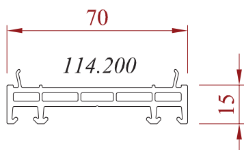
Elargisseur de 15 mm
