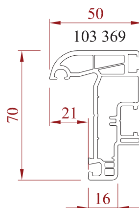
Battement de fenêtre
