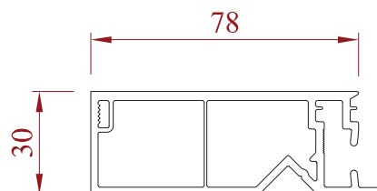
Tapée de 78 mm
