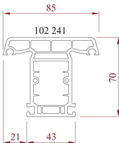
Traverse / Meneau de 85 mm
