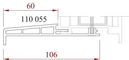
Pièce d'appui de 130 mm
