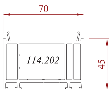
Elargisseur de 45 mm
