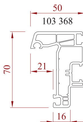
Battement de fenêtre
