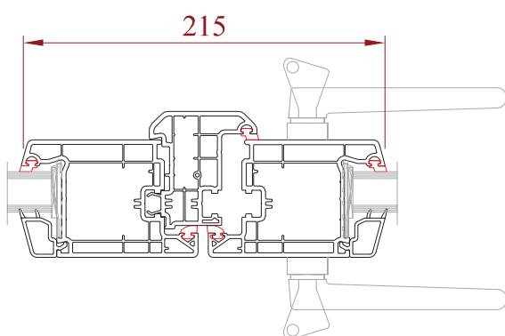
Battement rapporté 64 mm
