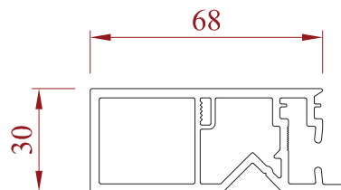
Tapée de 68 mm
