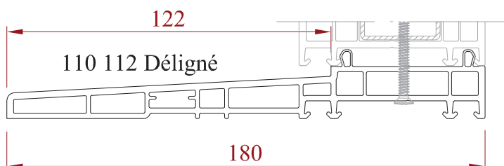
Pièce d'appui plate de 180 mm
