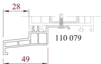
Pièce d'appui de 48 mm
