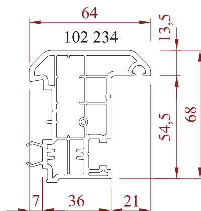
Battement rapporté 64 mm
