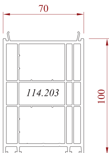
Elargisseur de 100 mm
