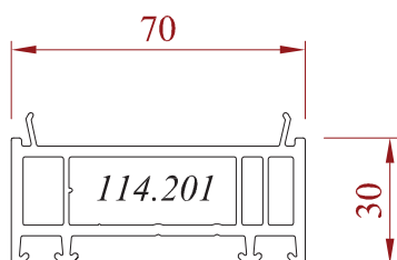
Elargisseur de 30 mm
