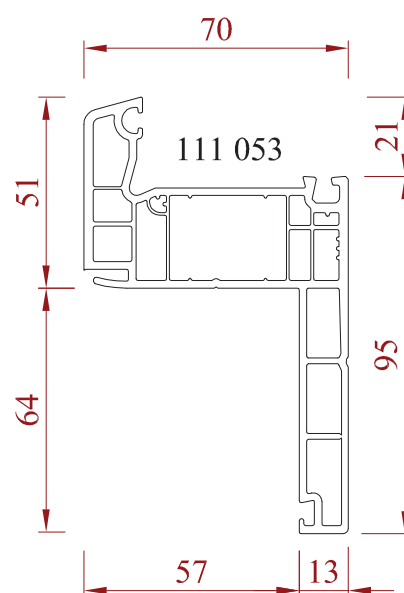
Dormant réno aile de 65 mm
