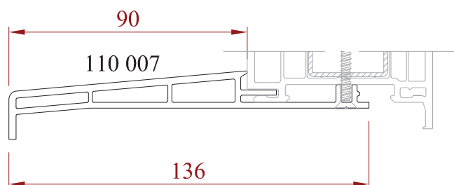
Pièce d'appui de 160 mm
