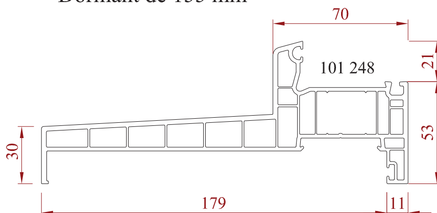
Dormant de 175 mm
