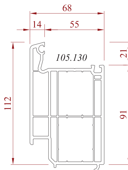
Elargisseur de 91 mm
