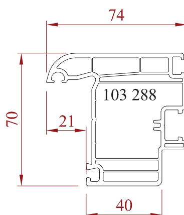
Battement de porte-fenêtre
