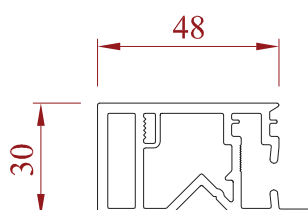
Tapée de 48 mm
