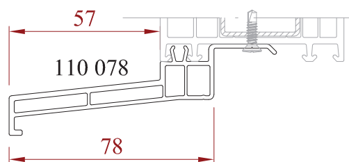
Pièce d'appui de 78 mm
