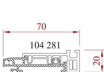
Seuil alu de 20 mm
