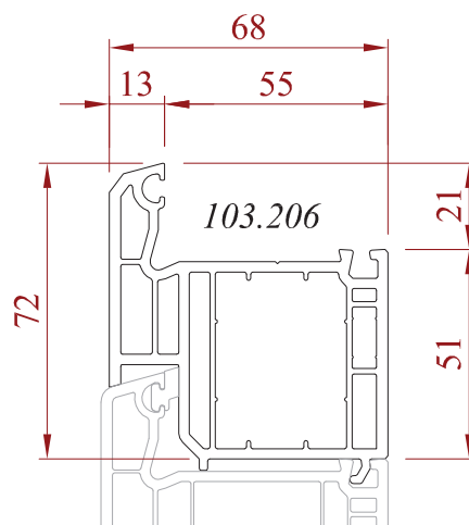
Elargisseur de dormant 72 mm
