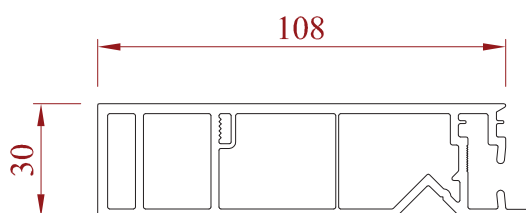
Tapée de 108 mm
