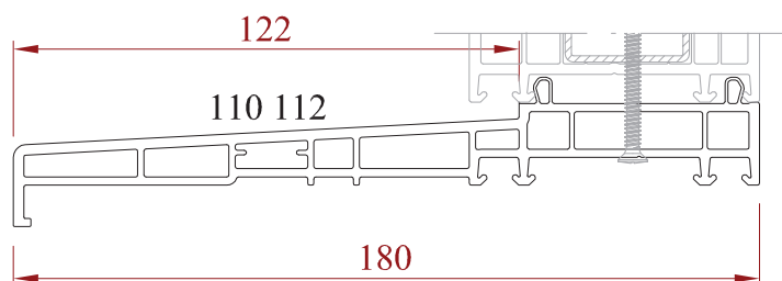
Pièce d'appui de 180 mm
