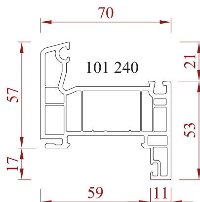
Dormant de 70 mm universel
