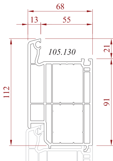
Elargisseur de dormant 112 mm
