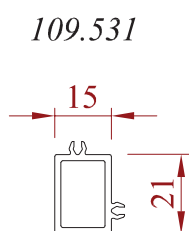
Compensateur 21x15mm
