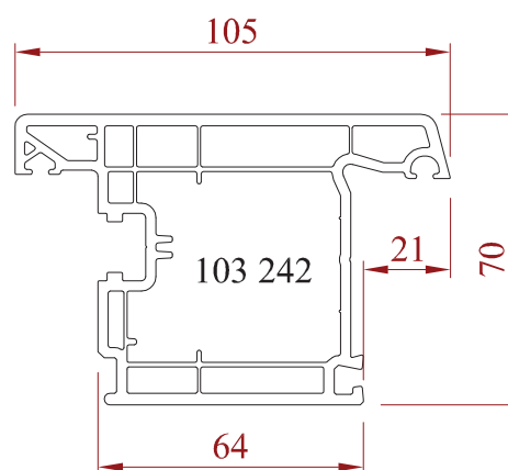
Ouvrant ouverture extérieur
