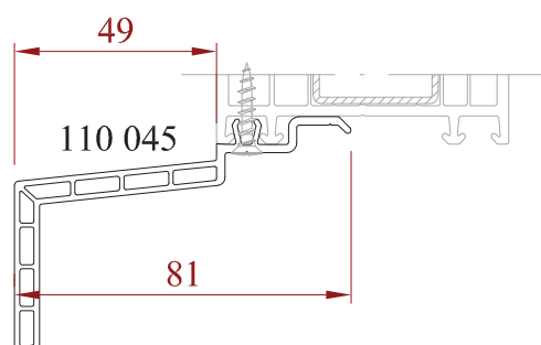
pièce d'appui de 50 x 48.5 mm
