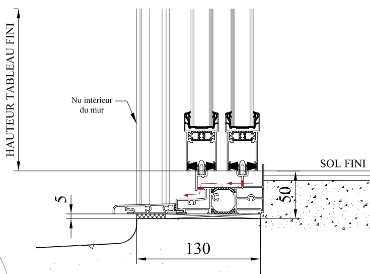
DETAIL PIECE D'APPUI
