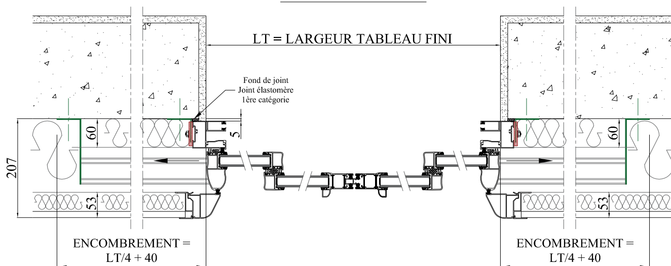
COUPE HORIZONTALE
