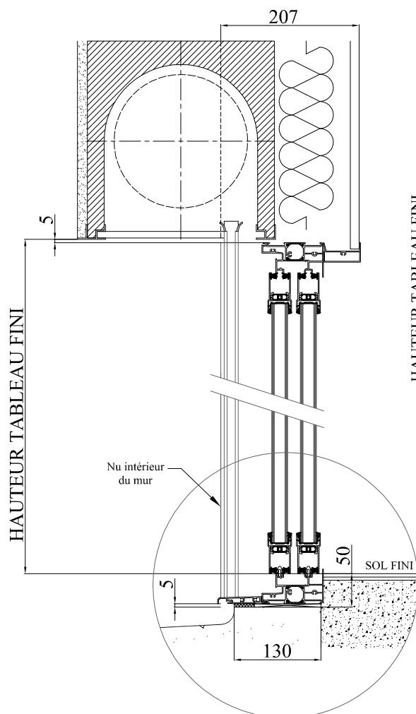
COUPE VERTICALE
