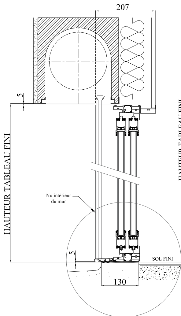
COUPE VERTICALE
