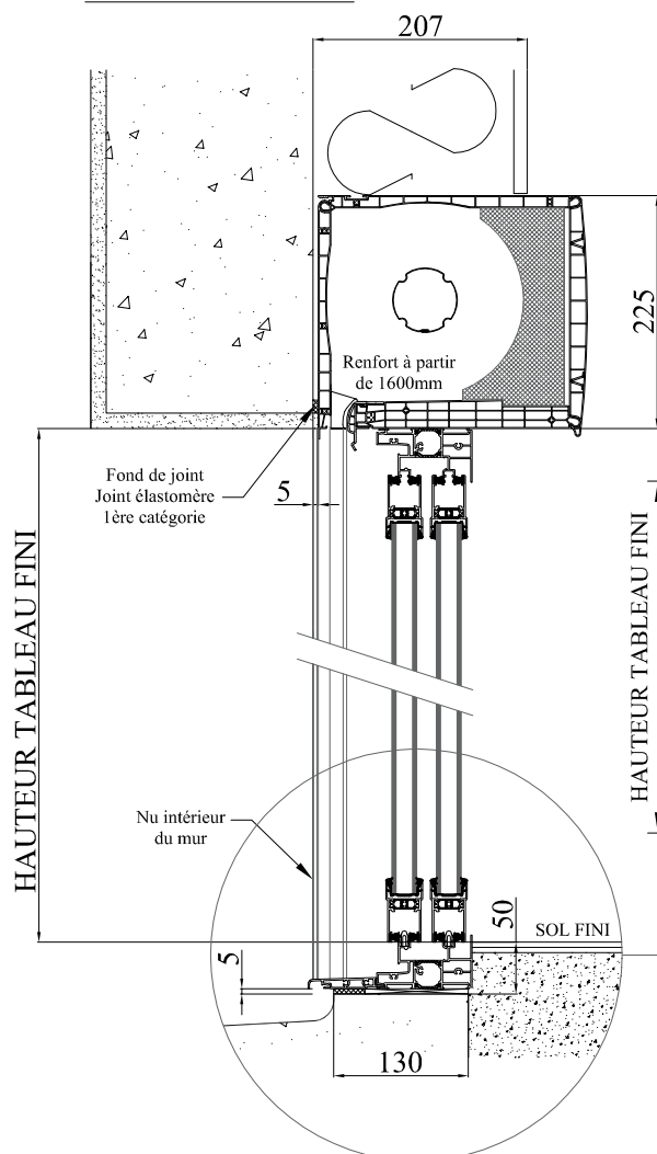
COUPE VERTICALE
