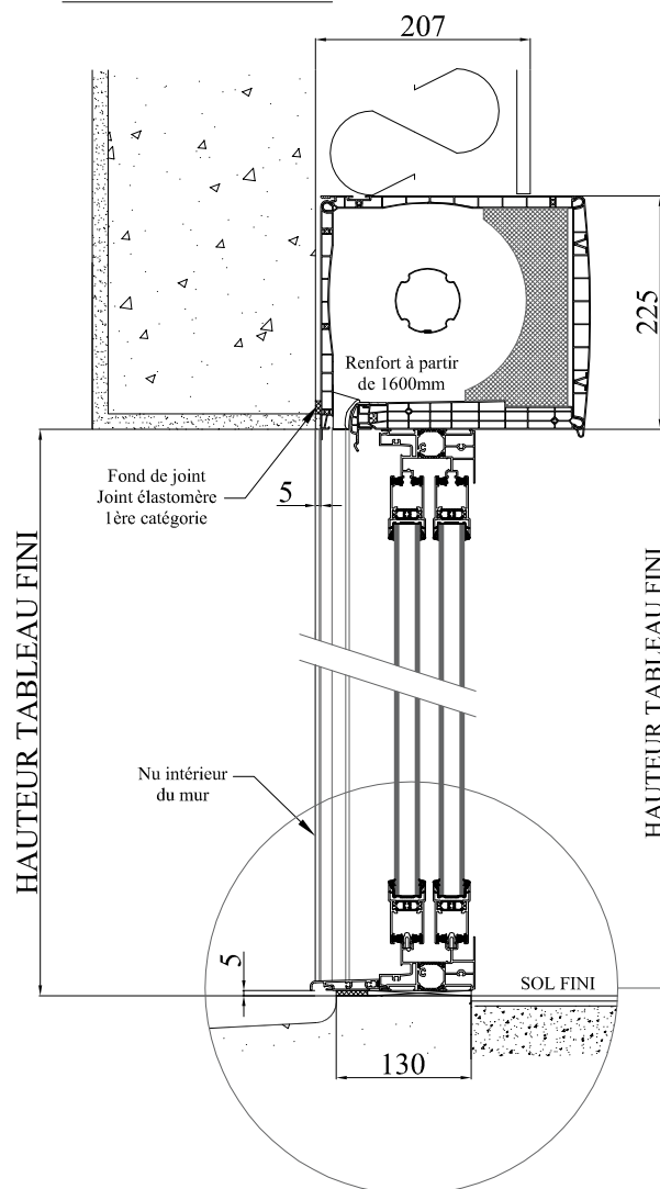
COUPE VERTICALE
