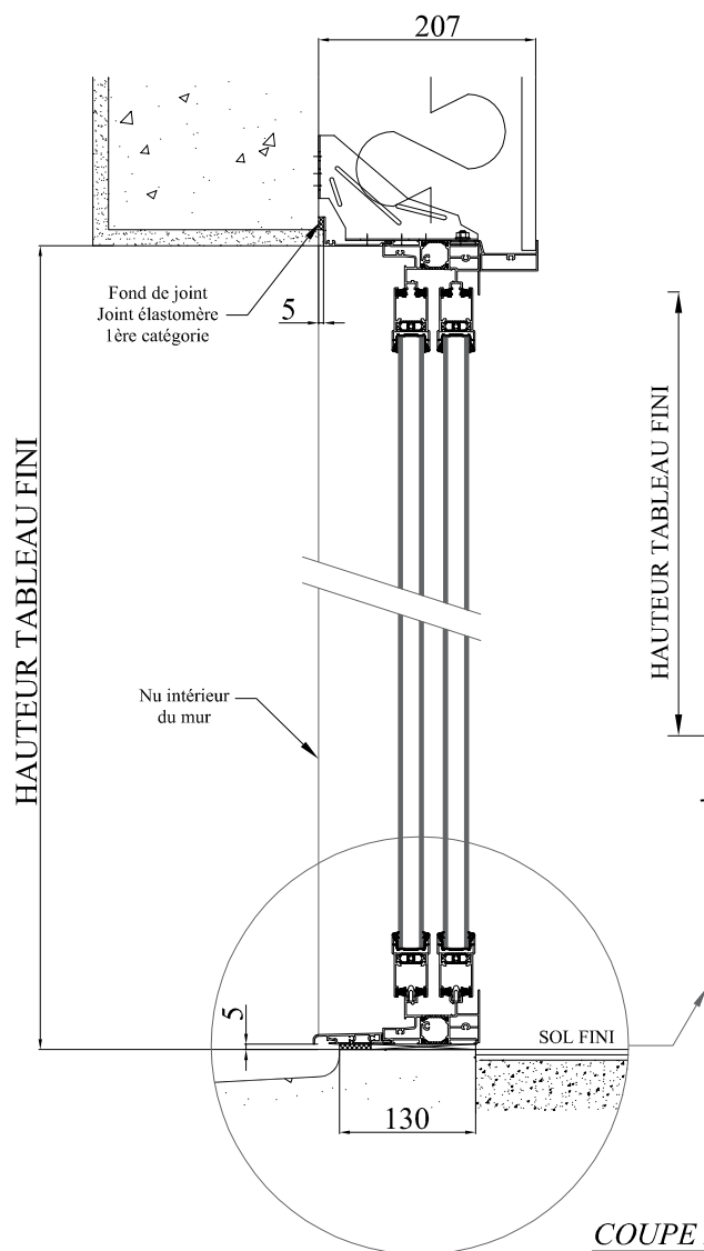
COUPE VERTICALE
