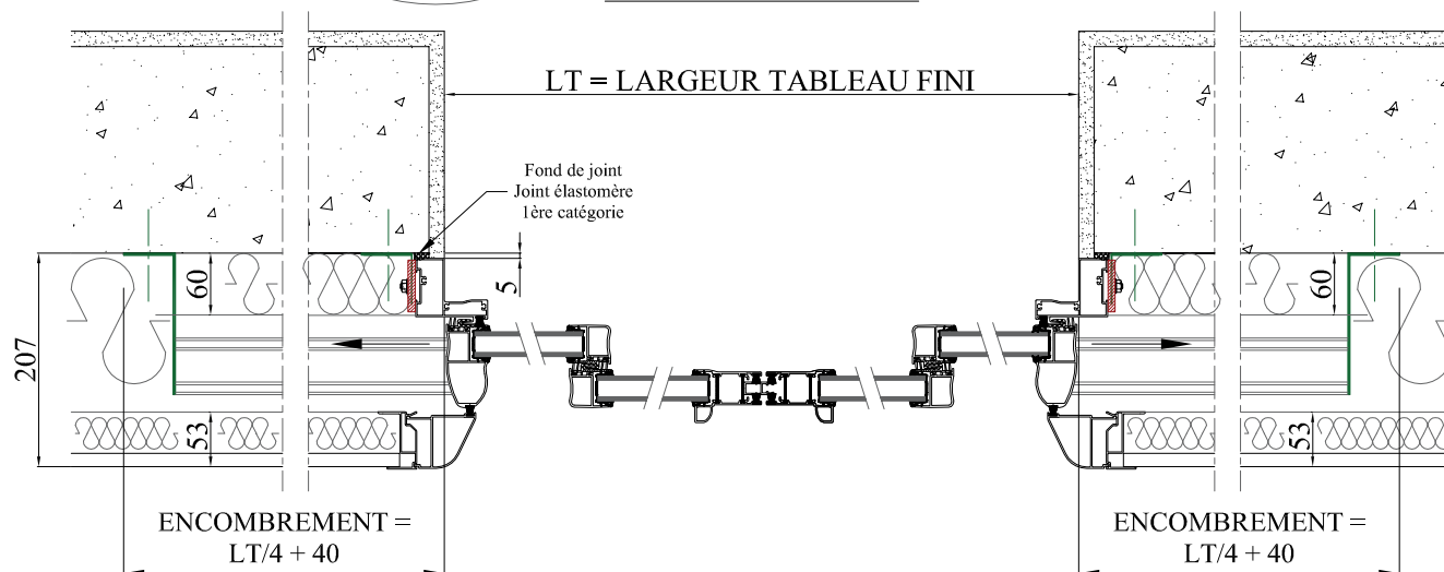
COUPE HORIZONTALE
