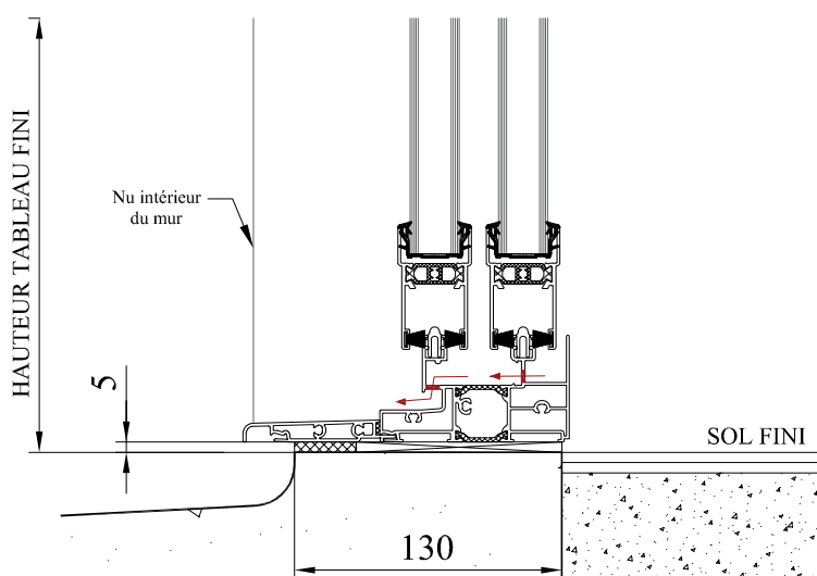
DETAIL PIECE D'APPUI
