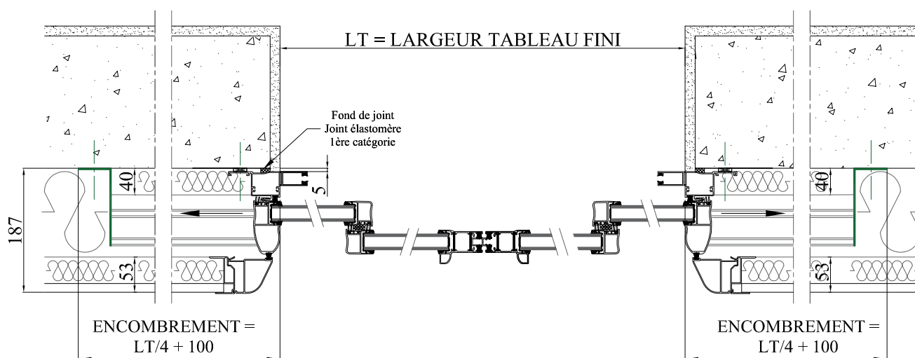
COUPE HORIZONTALE
