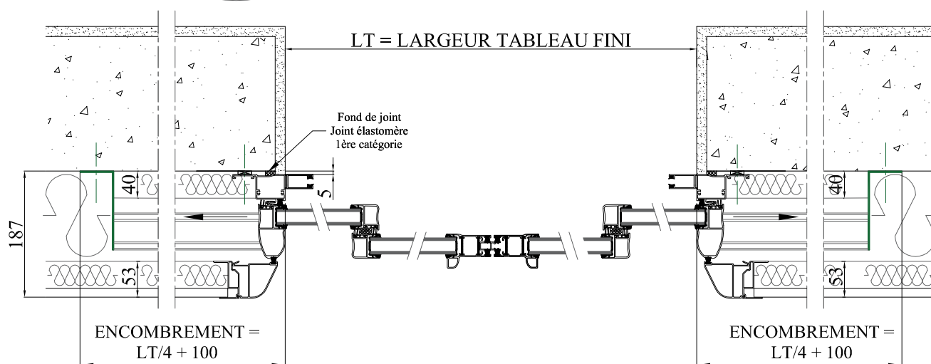
COUPE HORIZONTALE
