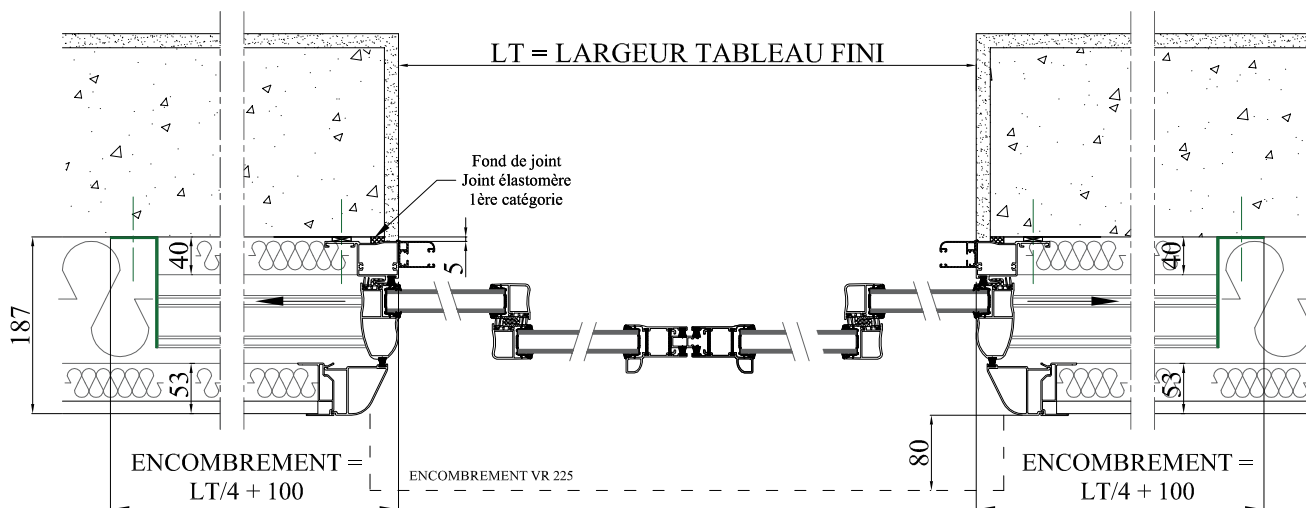
COUPE HORIZONTALE
