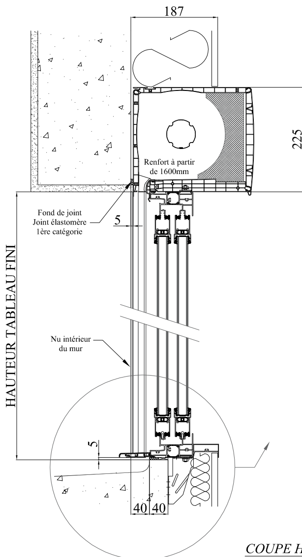
COUPE VERTICALE
