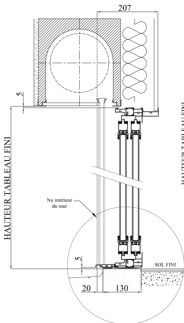
COUPE VERTICALE
