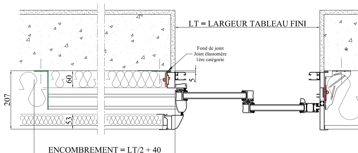
COUPE HORIZONTALE
