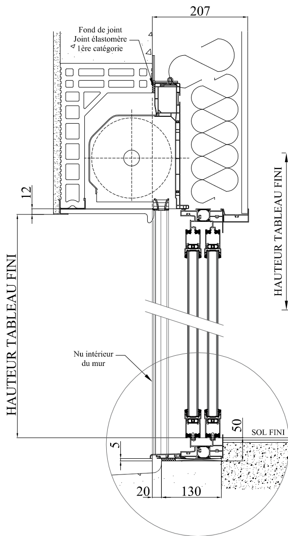
COUPE VERTICALE
