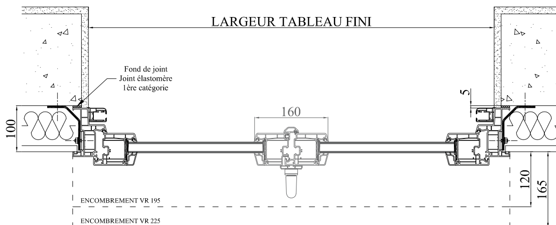
COUPE HORIZONTALE
