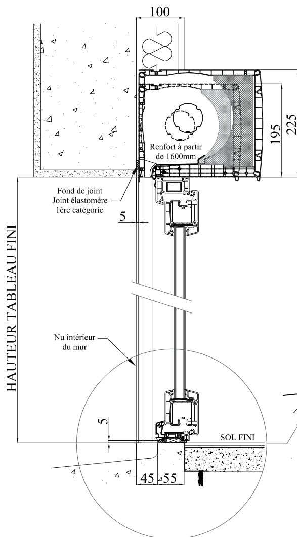
COUPE VERTICALE
