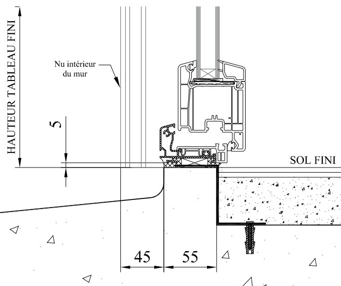
DETAIL PIECE D'APPUI
