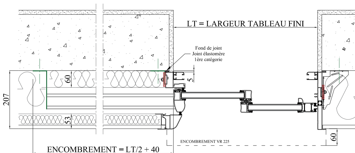
COUPE HORIZONTALE
