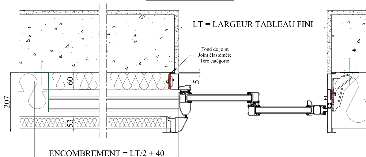
COUPE HORIZONTALE
