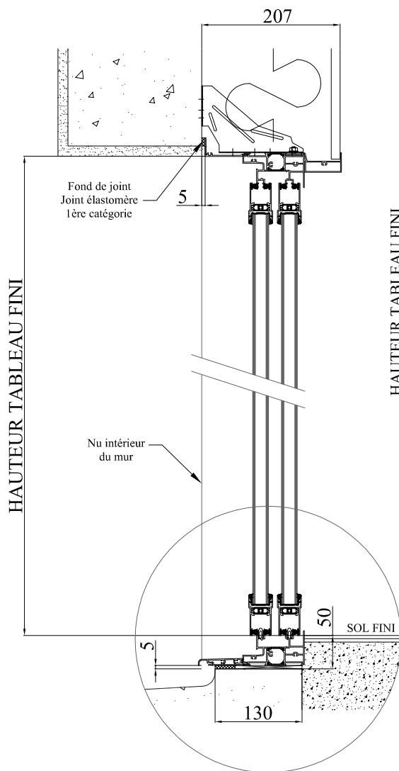
COUPE VERTICALE
