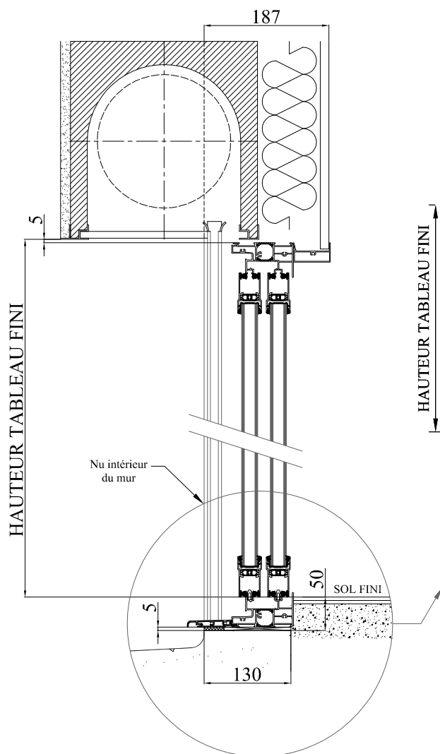
COUPE VERTICALE
