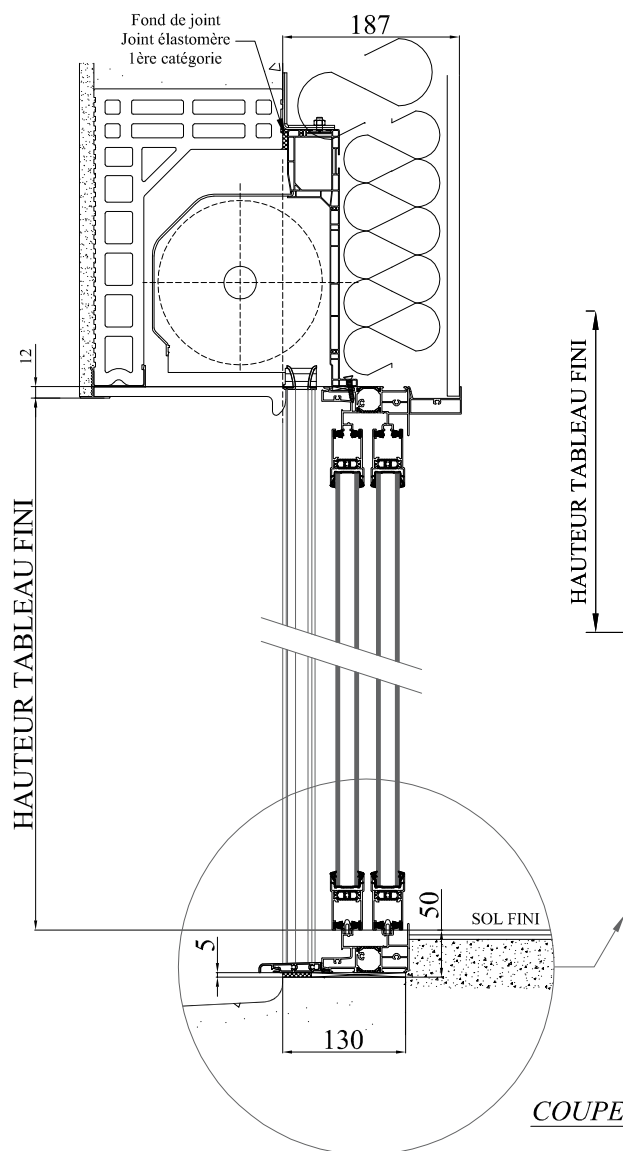
COUPE VERTICALE
