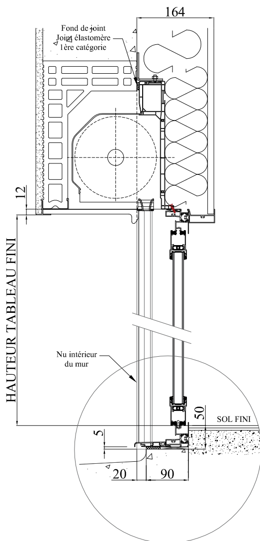
COUPE VERTICALE
