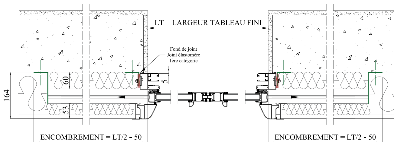
COUPE HORIZONTALE
