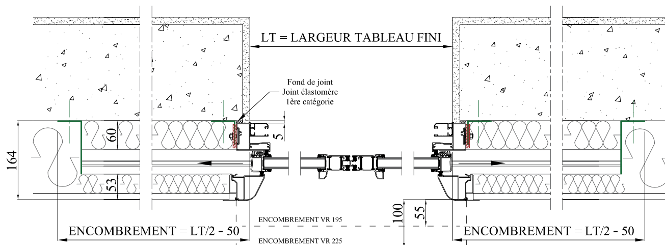
COUPE HORIZONTALE
