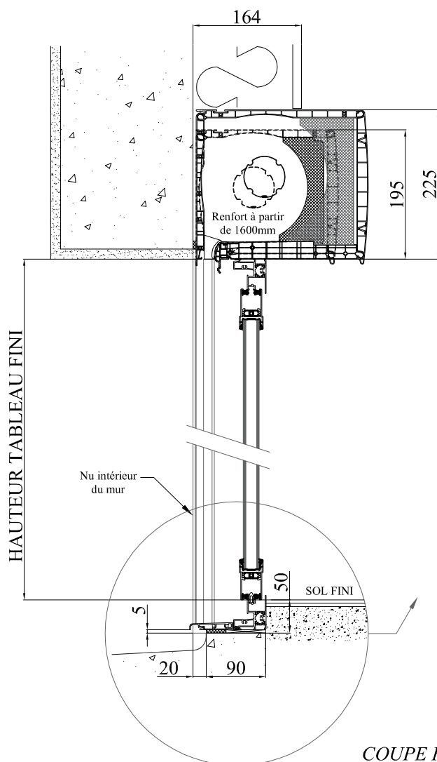
COUPE VERTICALE
