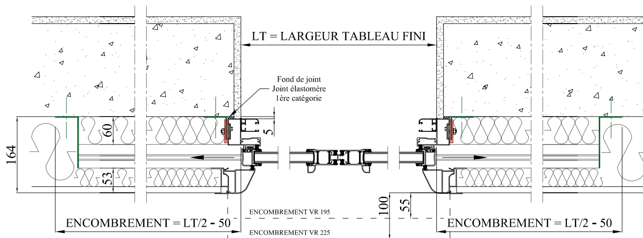
COUPE HORIZONTALE
