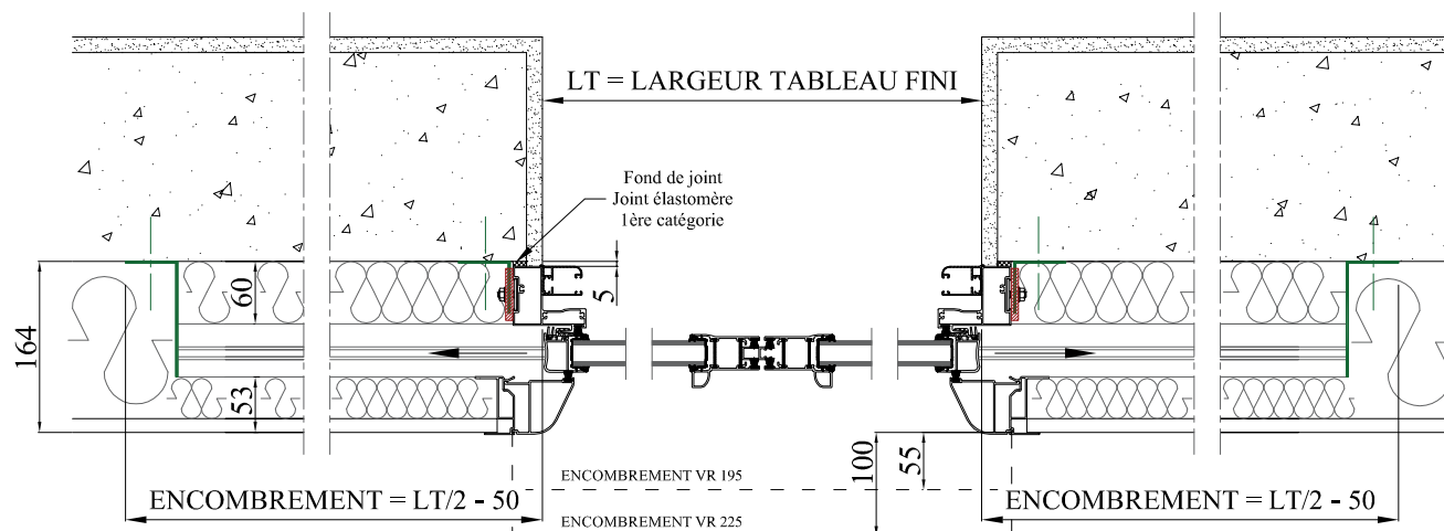
COUPE HORIZONTALE
