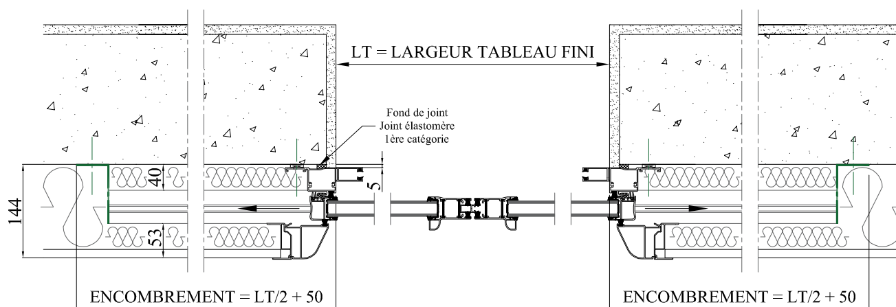
COUPE HORIZONTALE
