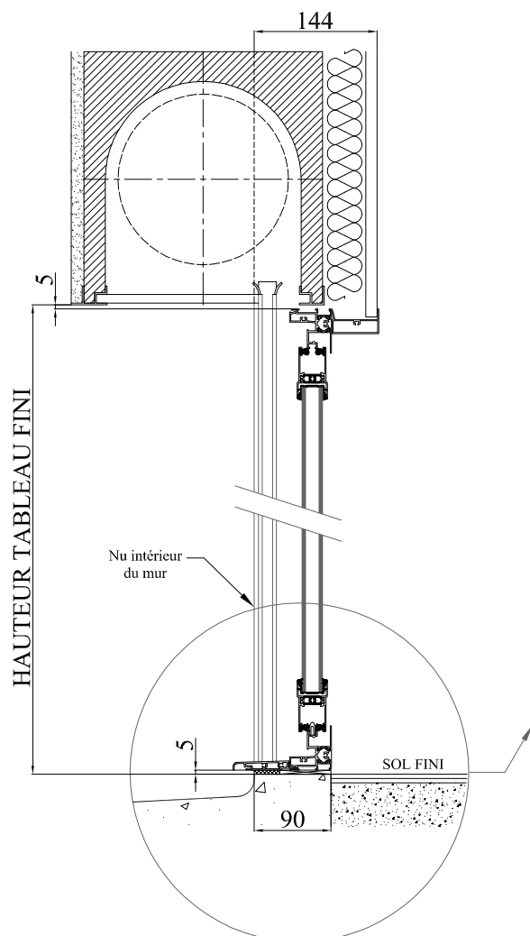
COUPE VERTICALE
