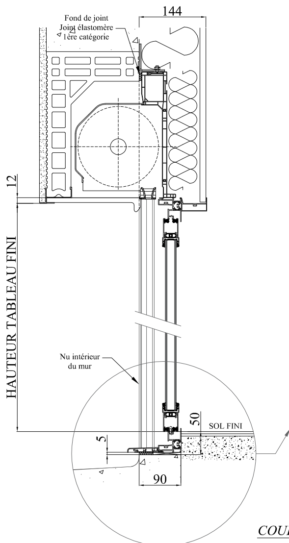
COUPE VERTICALE
