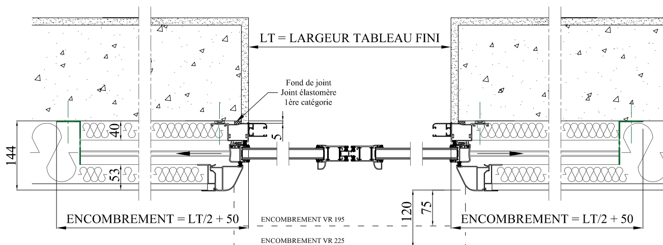
COUPE HORIZONTALE
