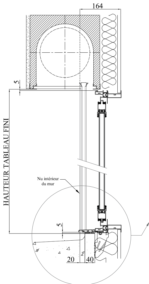
COUPE VERTICALE
