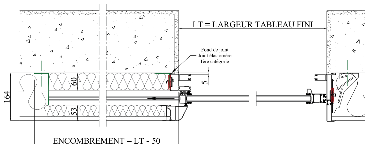
COUPE HORIZONTALE
