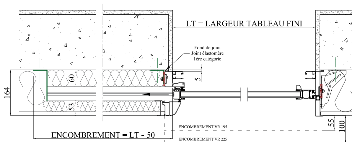
COUPE HORIZONTALE
