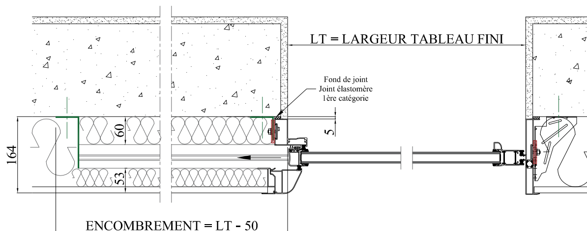
COUPE HORIZONTALE
