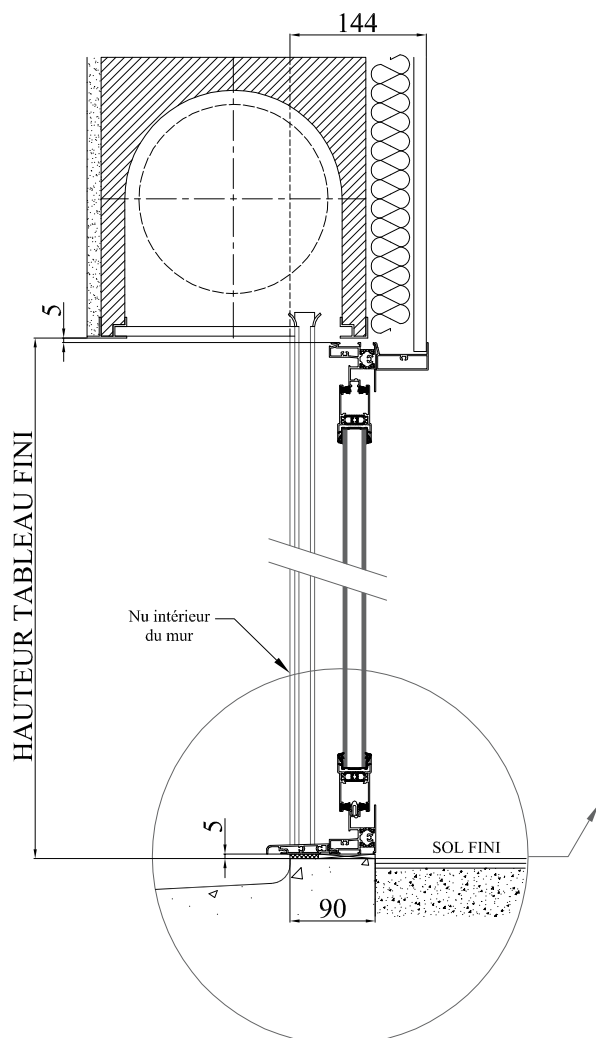
COUPE VERTICALE
