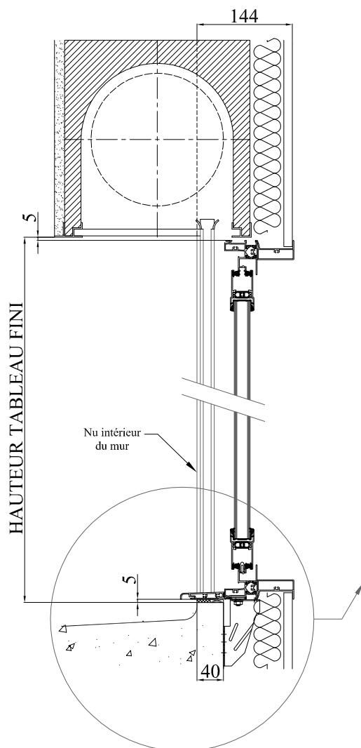
COUPE VERTICALE
