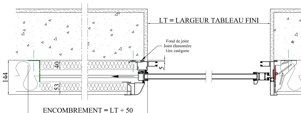
COUPE HORIZONTALE
