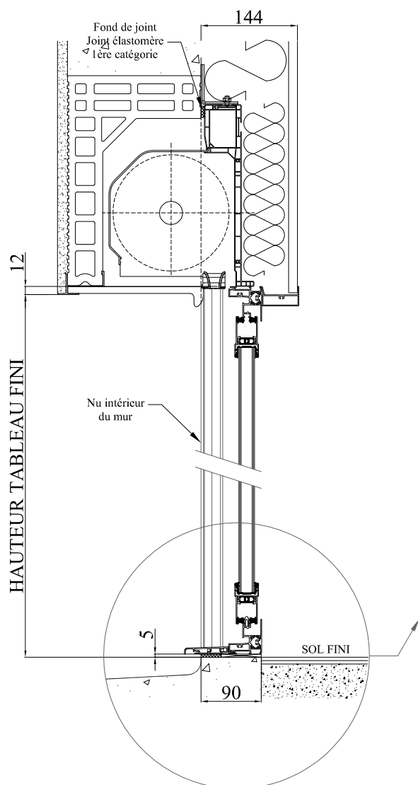
COUPE VERTICALE
