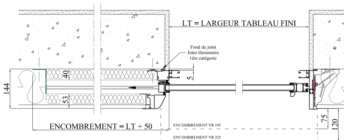
COUPE HORIZONTALE
