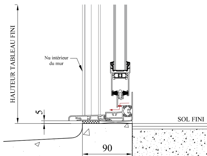
DETAIL PIECE D'APPUI
