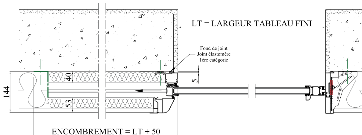
COUPE HORIZONTALE
