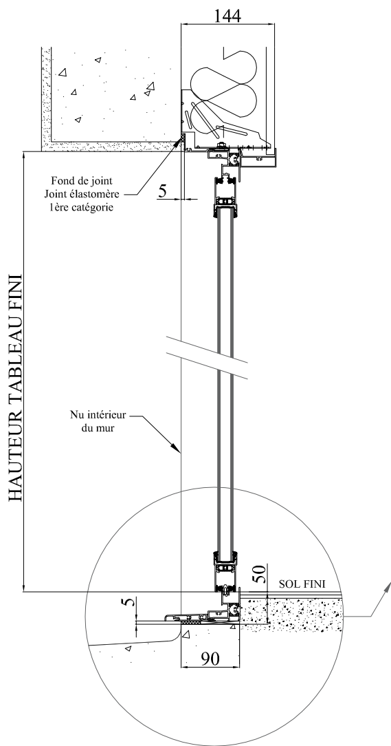
COUPE VERTICALE
