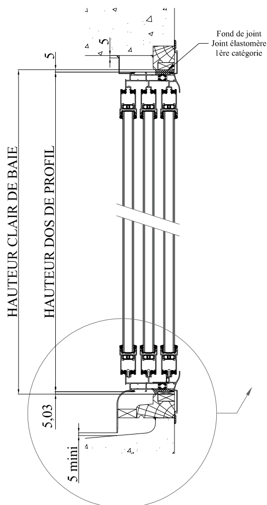
COUPE VERTICALE
