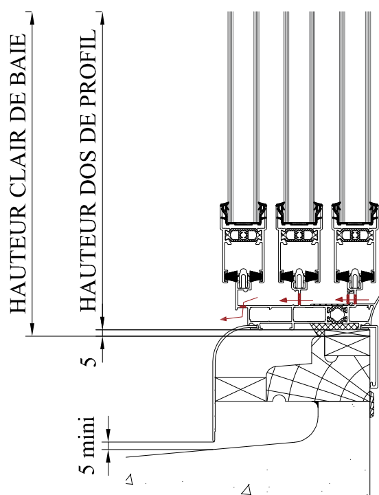
DETAIL PIECE D'APPUI
