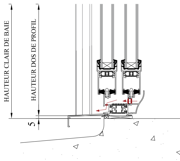
DETAIL PIECE D'APPUI
