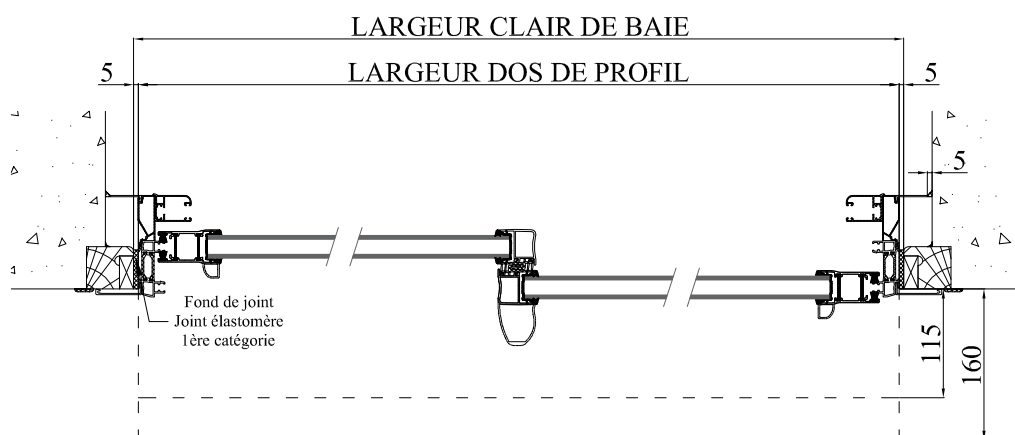
COUPE HORIZONTALE
