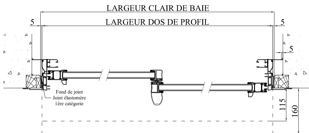
COUPE HORIZONTALE
