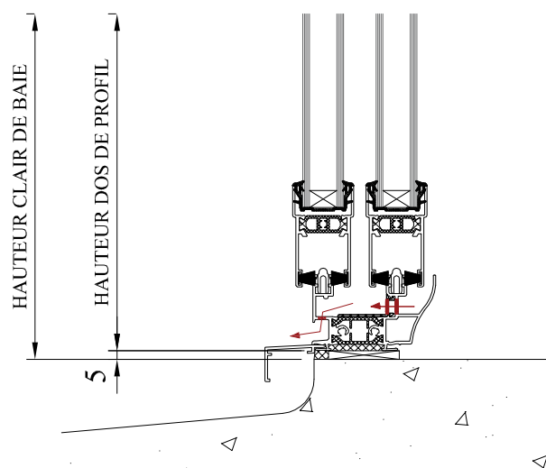
DETAIL PIECE D'APPUI
