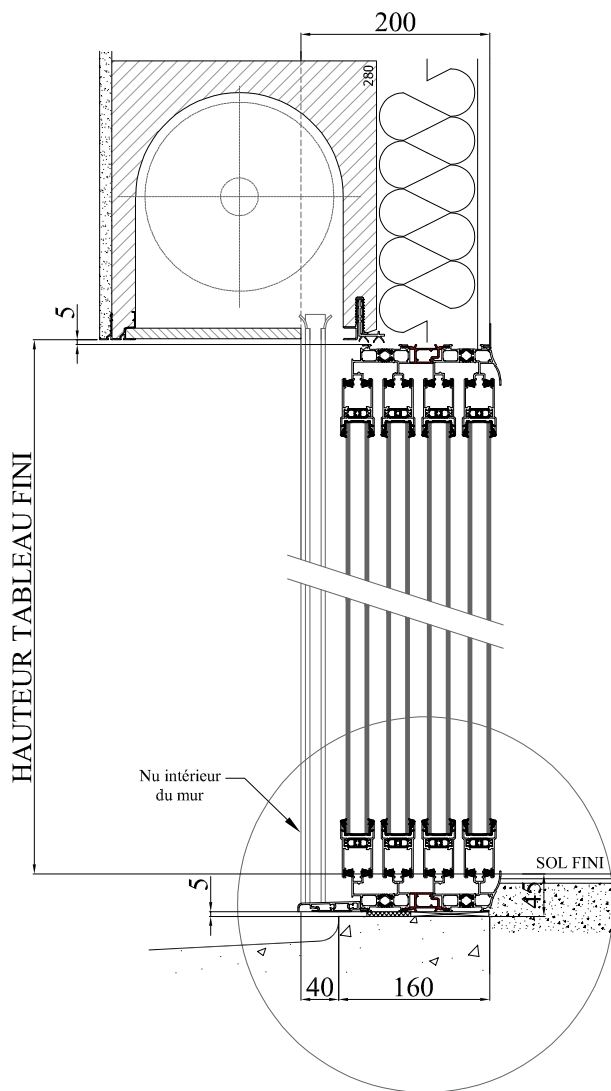
COUPE VERTICALE
