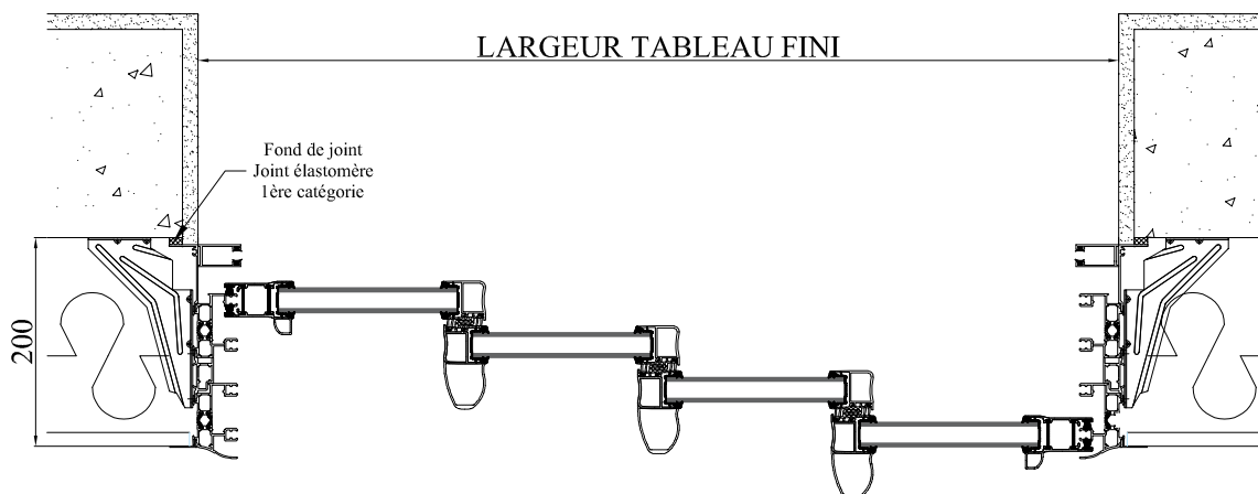
COUPE HORIZONTALE
