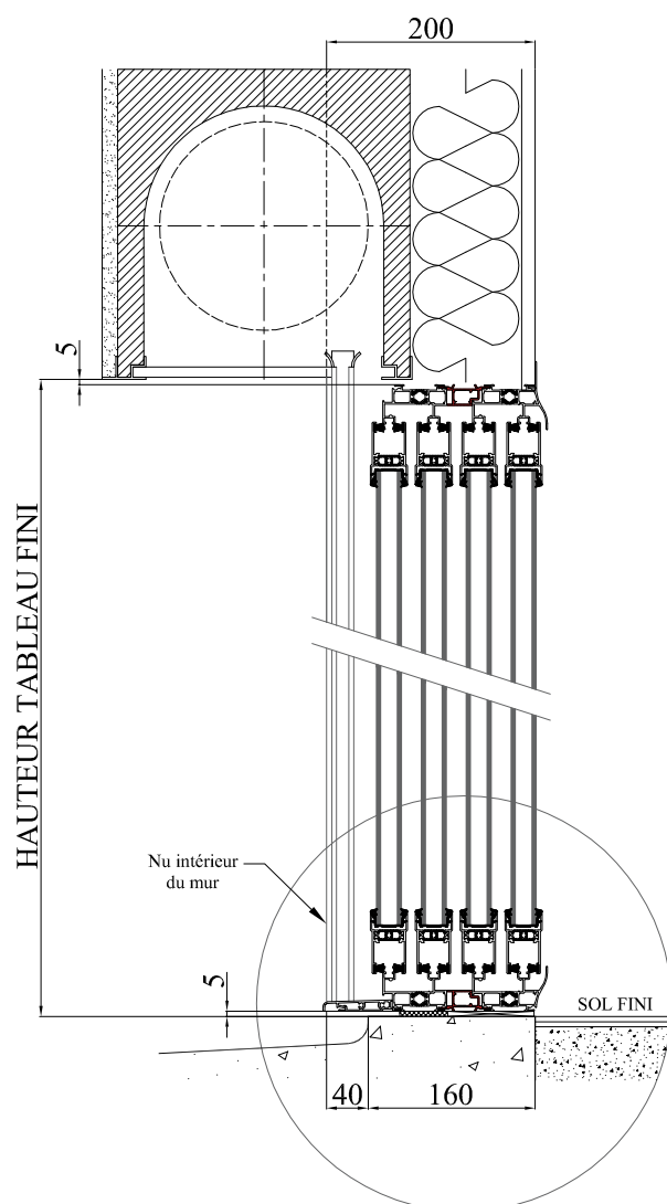
COUPE VERTICALE
