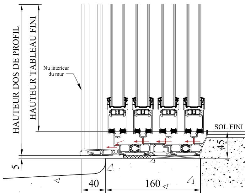
DETAIL PIECE D'APPUI
