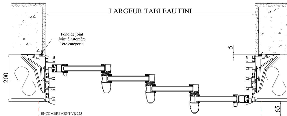
COUPE HORIZONTALE
