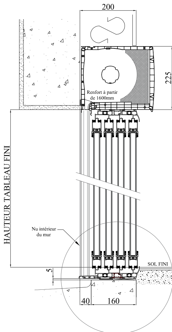
COUPE VERTICALE
