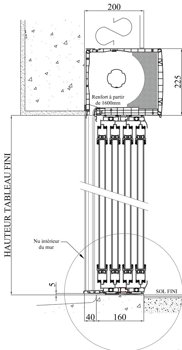
COUPE VERTICALE
