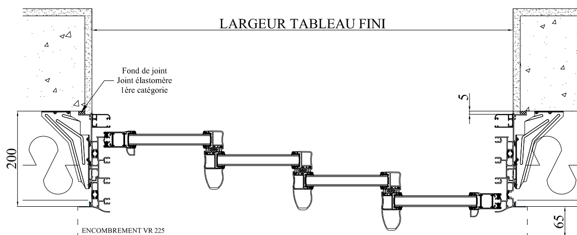
COUPE HORIZONTALE
