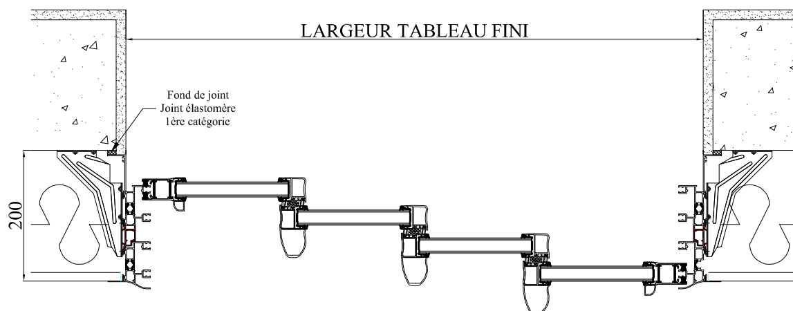
COUPE HORIZONTALE
