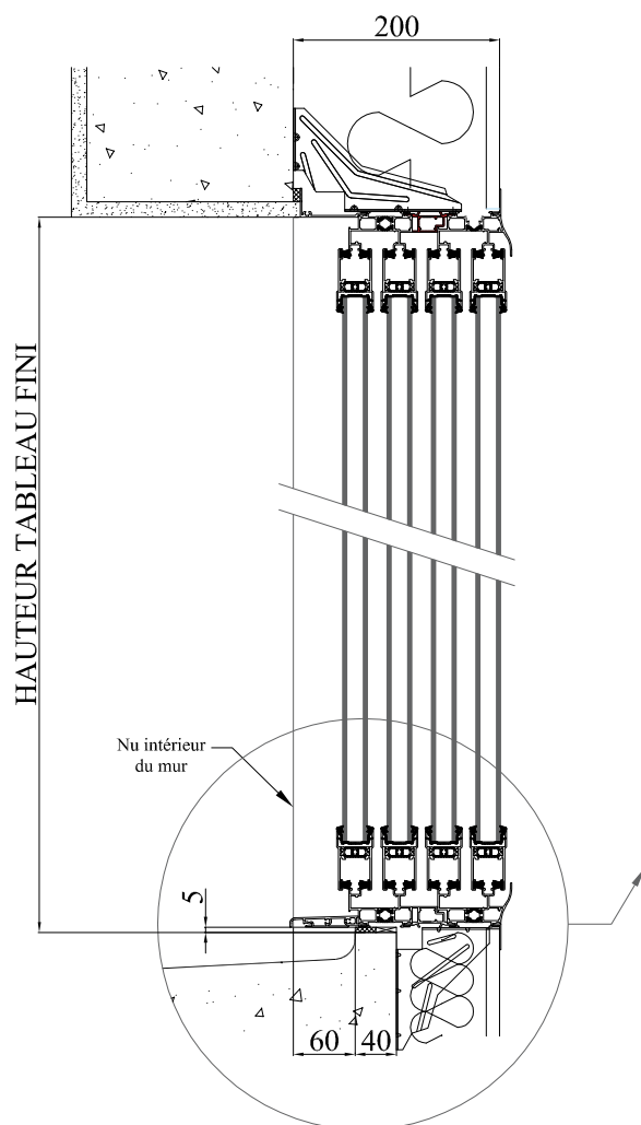
COUPE VERTICALE
