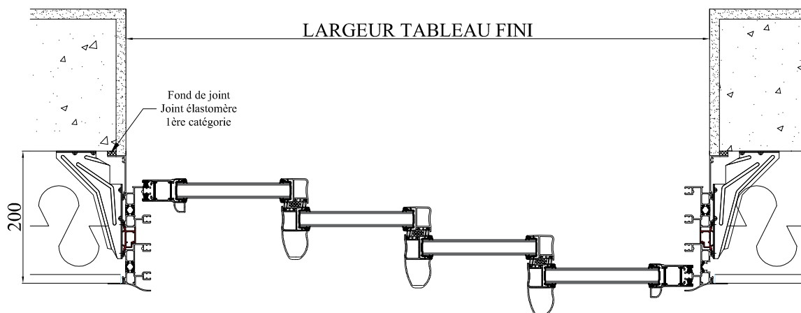
COUPE HORIZONTALE
