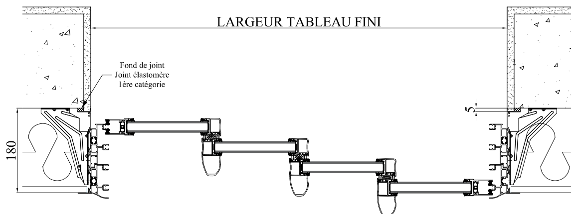
COUPE HORIZONTALE
