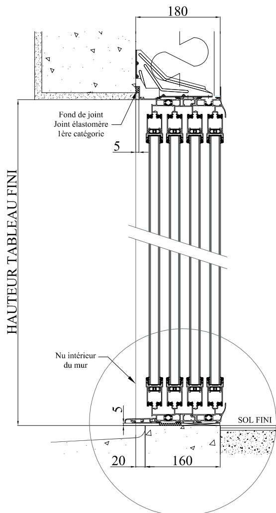
COUPE VERTICALE
