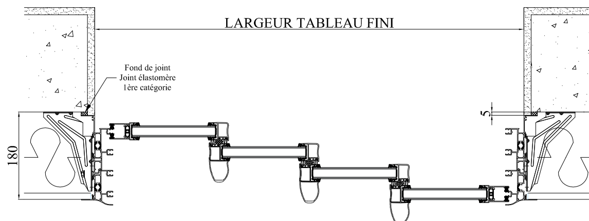
COUPE HORIZONTALE
