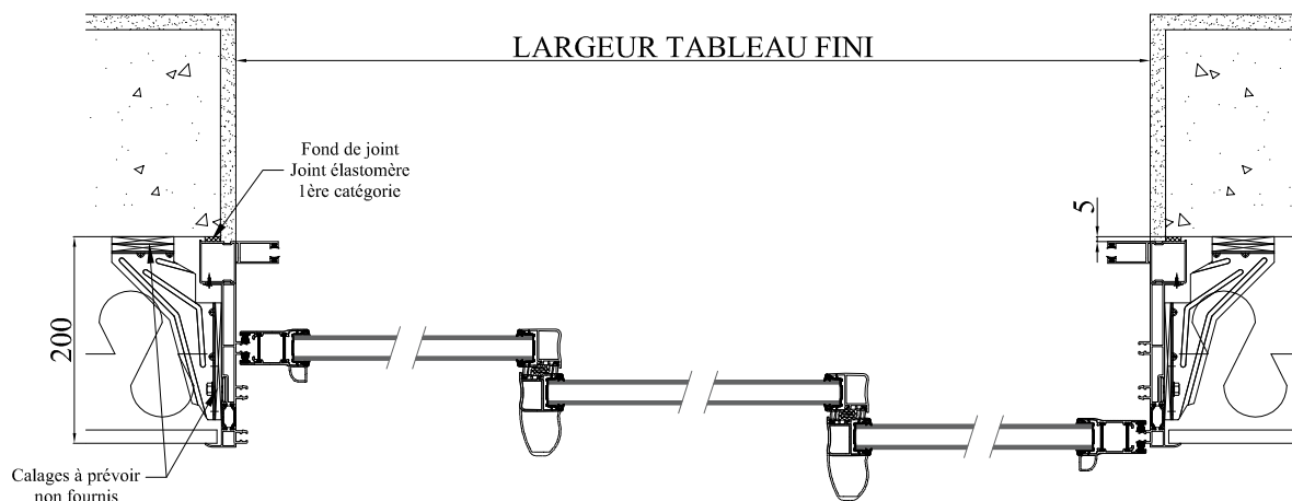
COUPE HORIZONTALE
