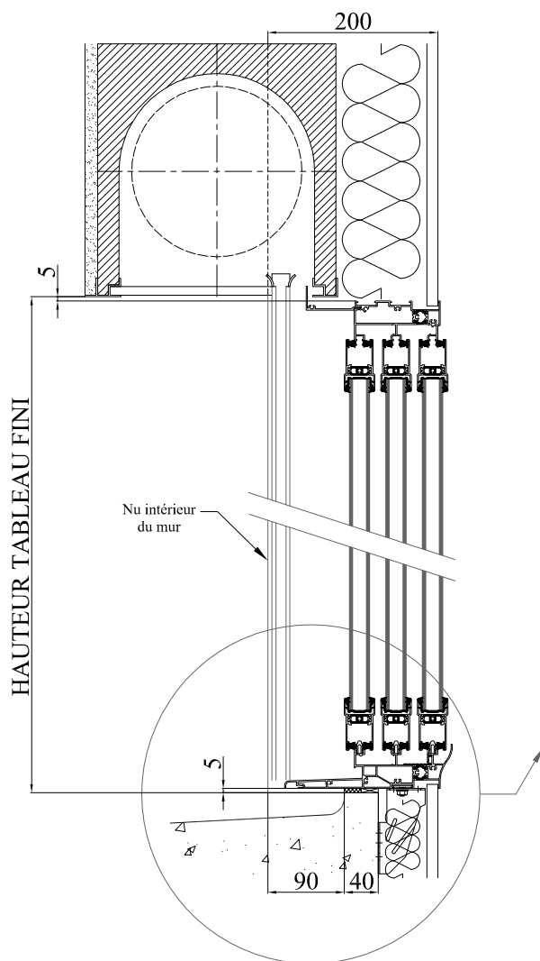
COUPE VERTICALE
