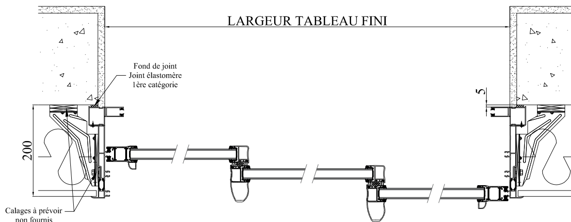
COUPE HORIZONTALE
