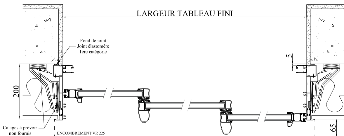
COUPE HORIZONTALE
