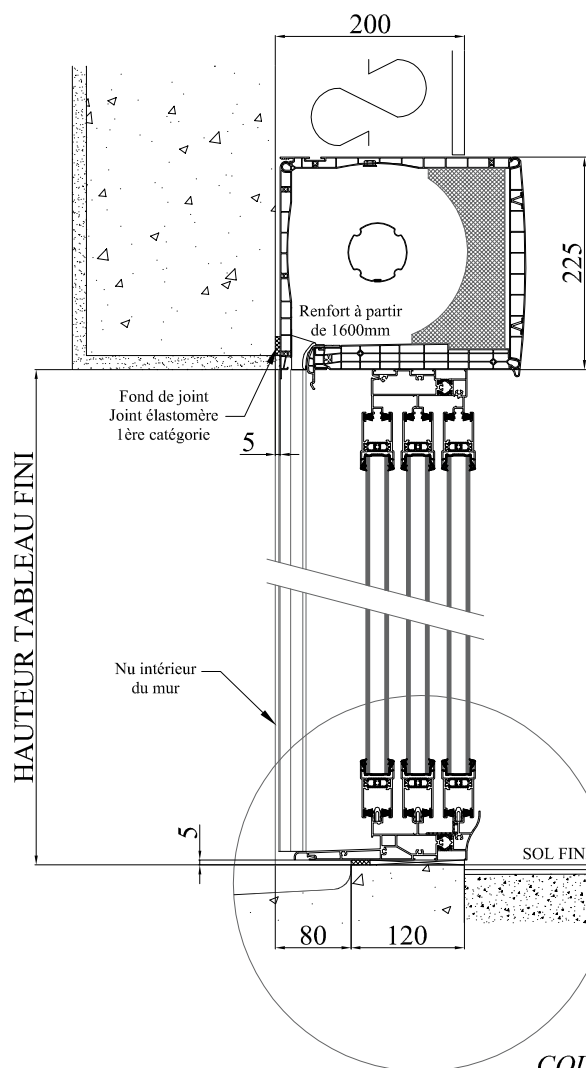
COUPE VERTICALE
